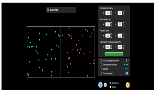
Диффузия
