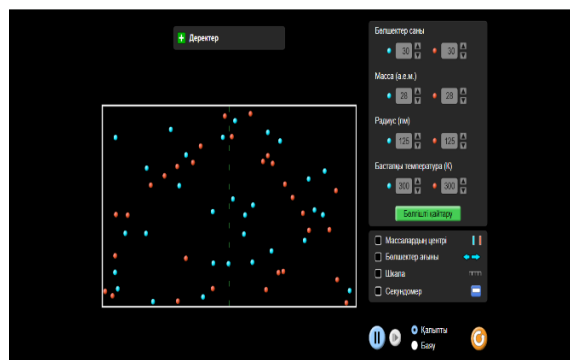
Диффузия
